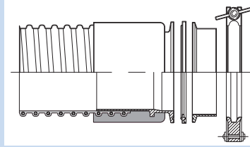
TRI-Clamp Kupplung passend zu Stutzen nach DIN 32676
