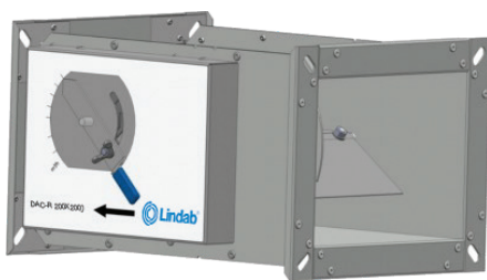
DAC-R ohne Isolierung
