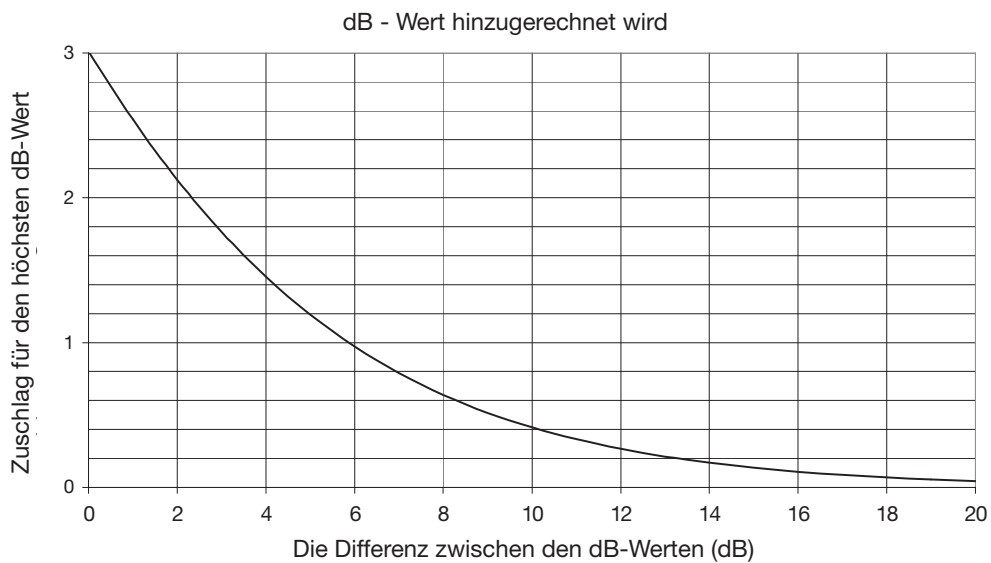
Abbildung 17: Addition von Schallpegeln (logarithmische Addition von Schalleistungspegel oder Schalldruckpegel).
