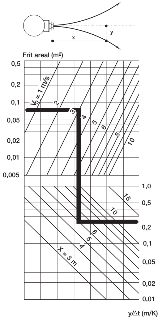
Abbildung 3: Nicht-isotherme Zuluft.
