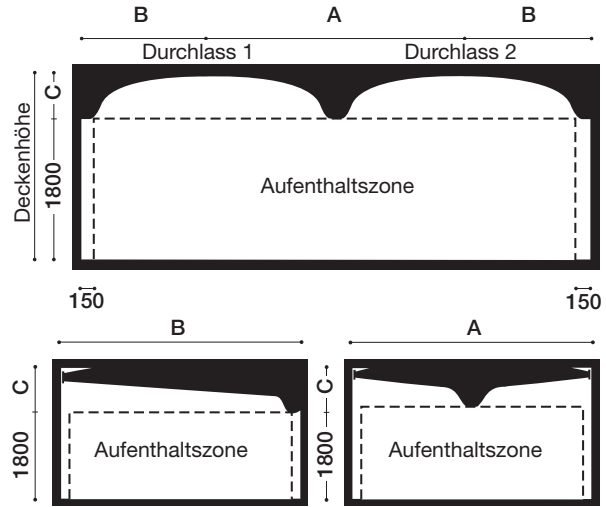
Abb. 1: Gegeneinander gerichtete Zuluftdurchlässe.
