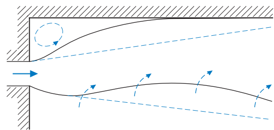
Bild.10 Luftströmung mit Coanda-Effekt.
