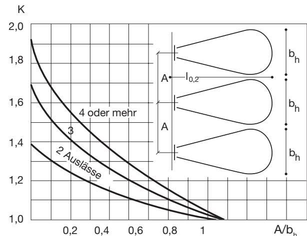
Abb. 2: Parallel gerichtete Zuluftdurchlässe.
