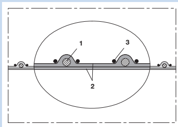
Silikonschlauch, doppelagig, dicht (bis +280°C)
