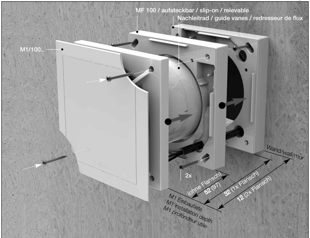
Alle Maße in mm / All dimensions in mm / Dimensions en mm
