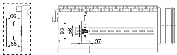
Trafo 20VA
