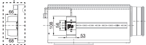
Trafo 20VA
